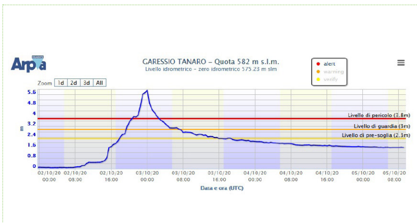
Idrometro Garesio (CN) – Fiume Tanaro - Livello max raggiunto = 5,93 m.
